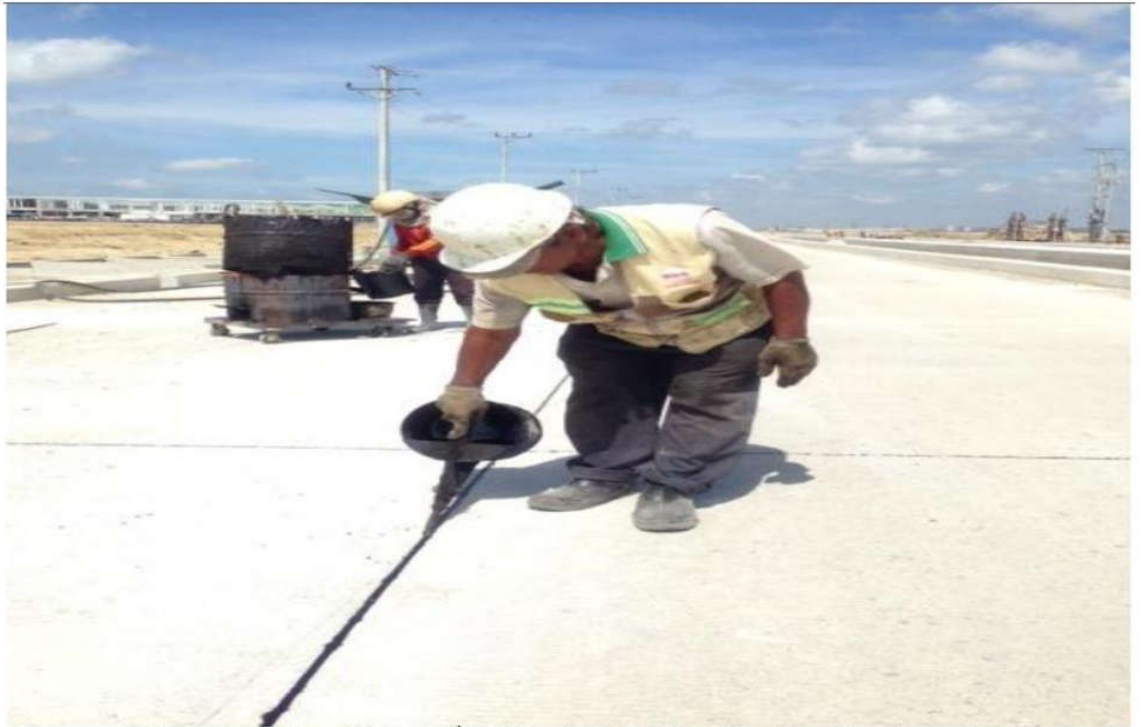
Thi công trám khe bê tông bằng Mastic MDS-2HK do Viện Khoa học và Công nghệ hàng không nghiên cứu và sản xuất tại KCN Phú Mỹ 3
